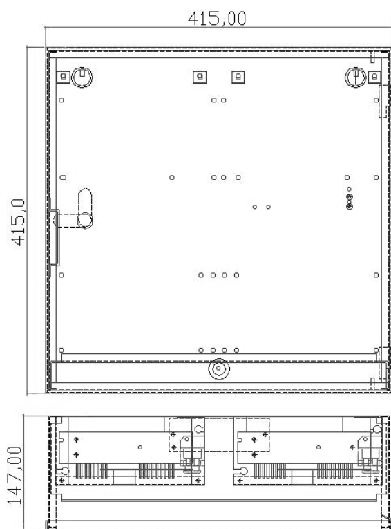
Рисунок 1.1 – Внешний вид ИБП Штиль PS4802E
